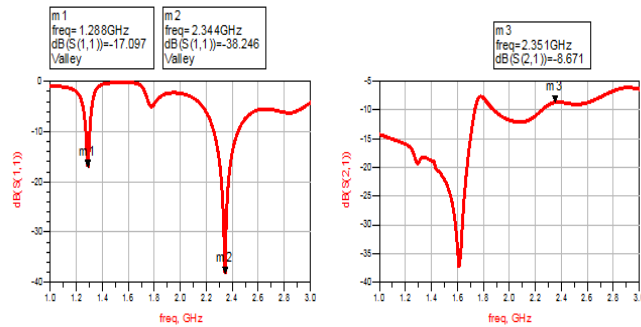
Fig. 5 (e) S-Parameters
