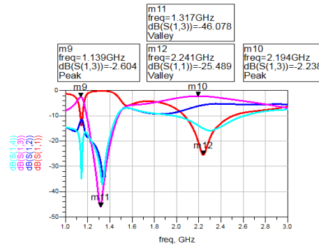
Fig. 8 S-Parameters
